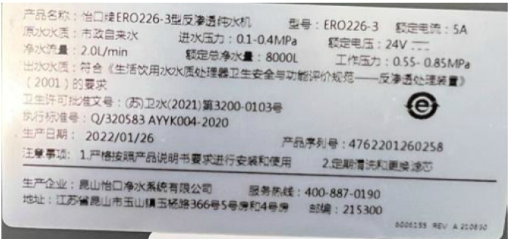
ERO226-3（铭牌）
